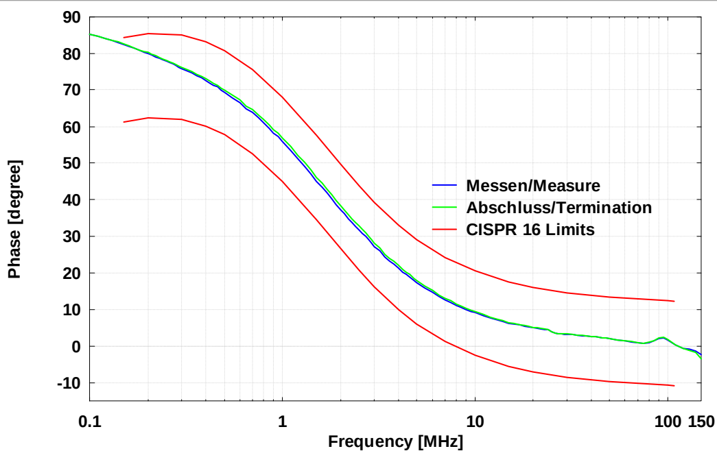
Abb. 5: Phase der Impedanz an den Prüflingsklemmen (Kalibrieradapter KA 8125 erforderlich), BNC mit 50 \Omega Abschluss, Speiseklemmen kurzgeschlossen
