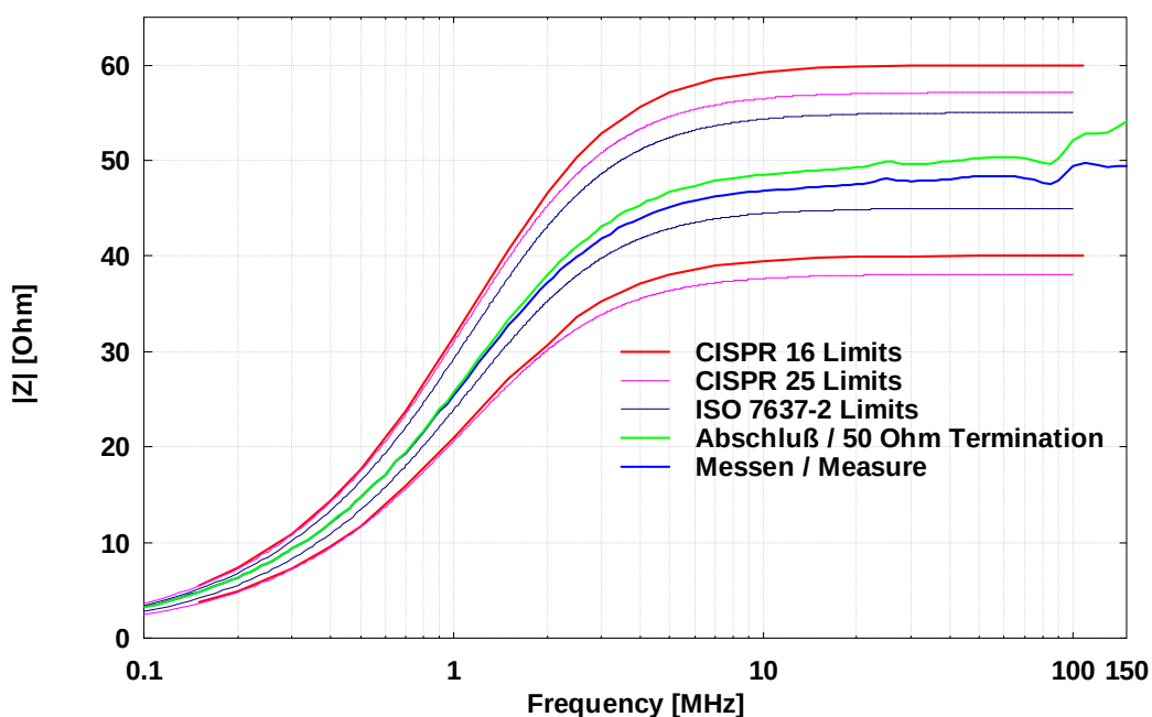
Abb. 4: Betrag der Impedanz an den Prüflingsklemmen (Kalibrieradapter KA 8125 erforderlich), BNC mit 50 \Omega Abschluss, Speiseklemmen kurzgeschlossen
